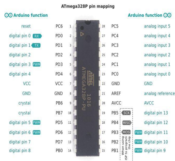
Fig. 2: Pin Diagram.
